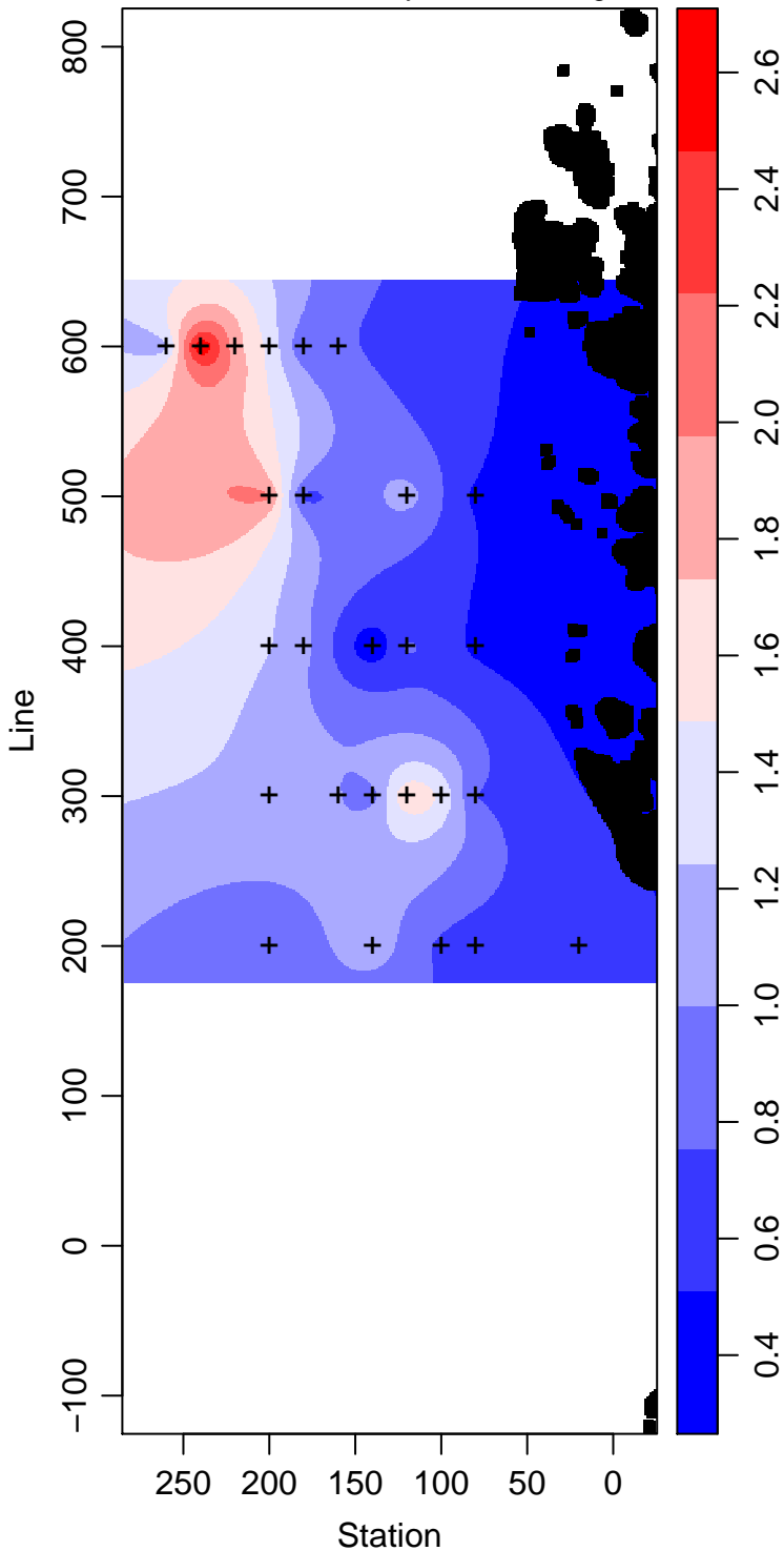
LMG04-01_75_Primary.Production mg m -3
