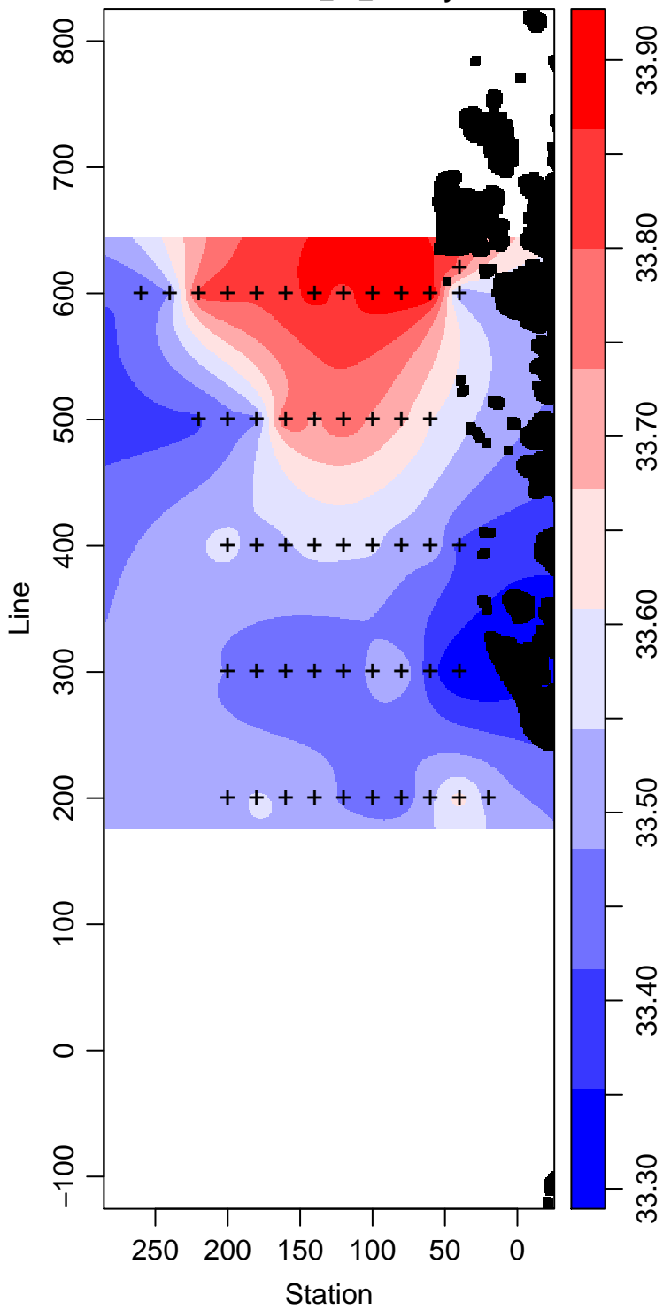
LMG04-01_15_Salinity
