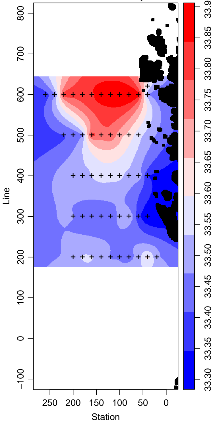
LMG04-01_1_Salinity
