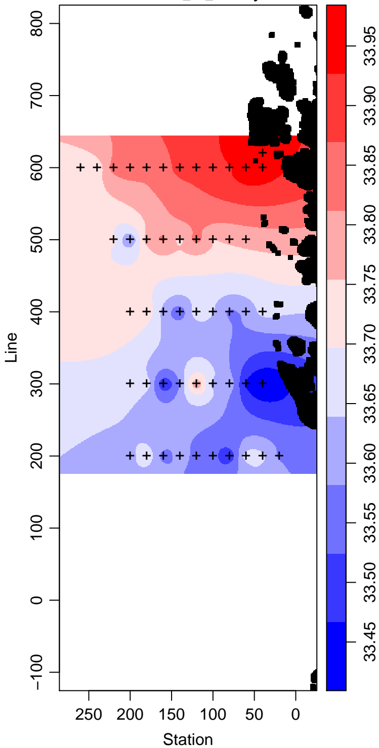
LMG04-01_35_Salinity
