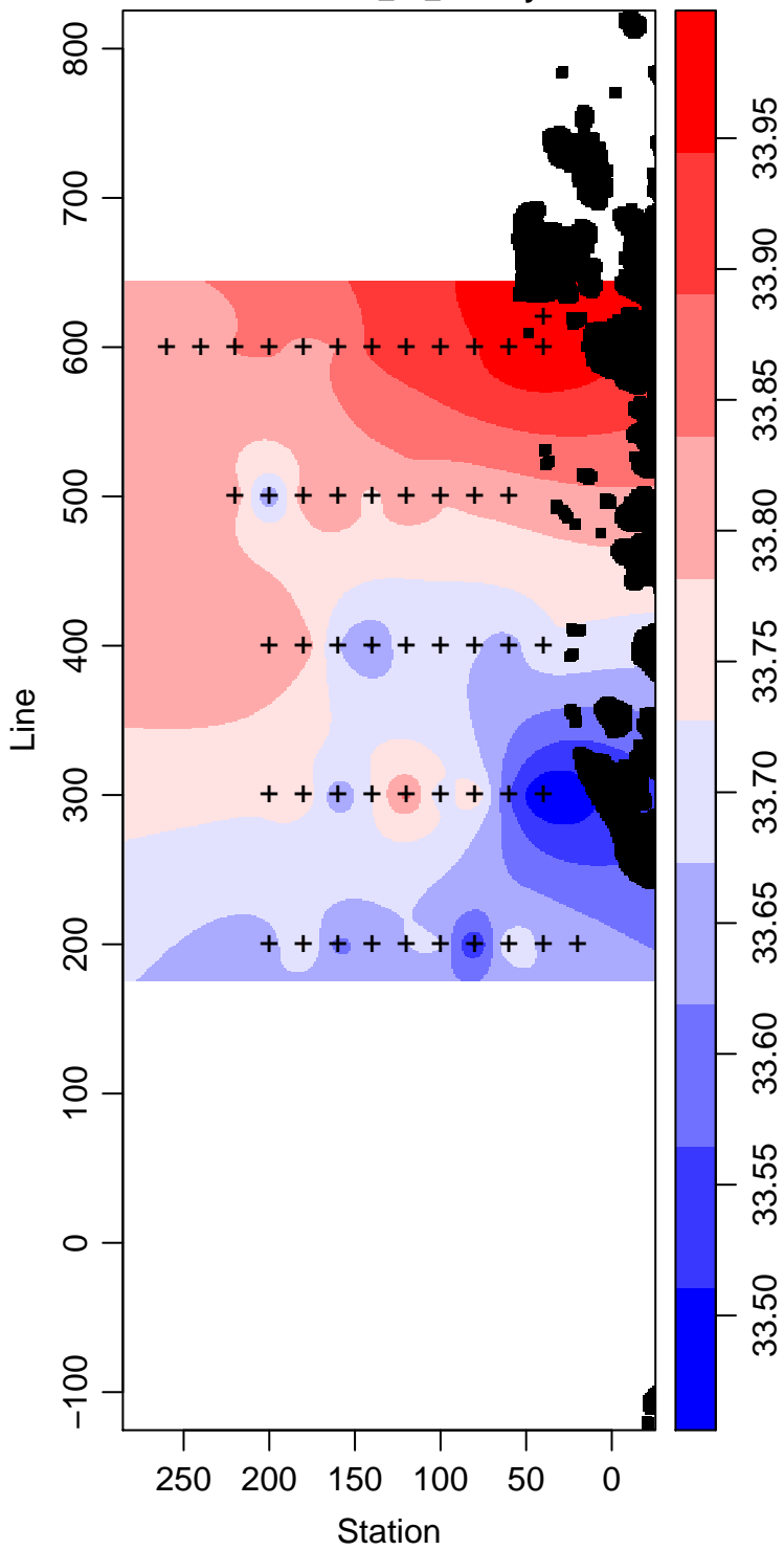
LMG04-01_40_Salinity
