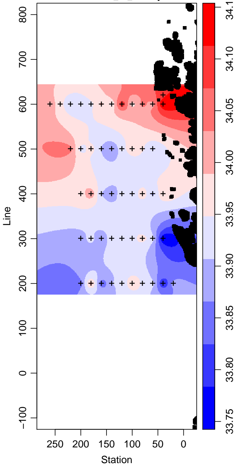
LMG04-01_65_Salinity
