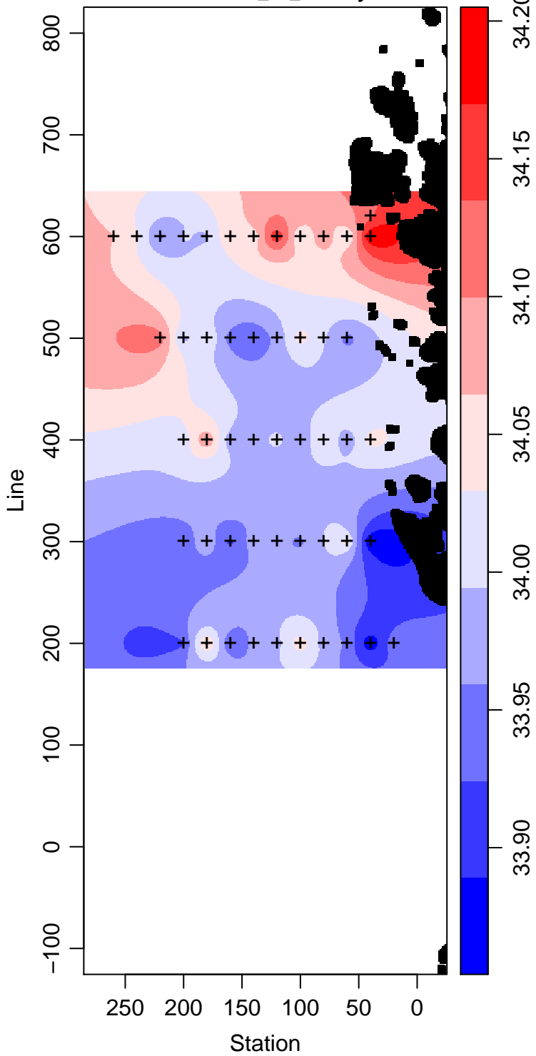
LMG04-01_75_Salinity
