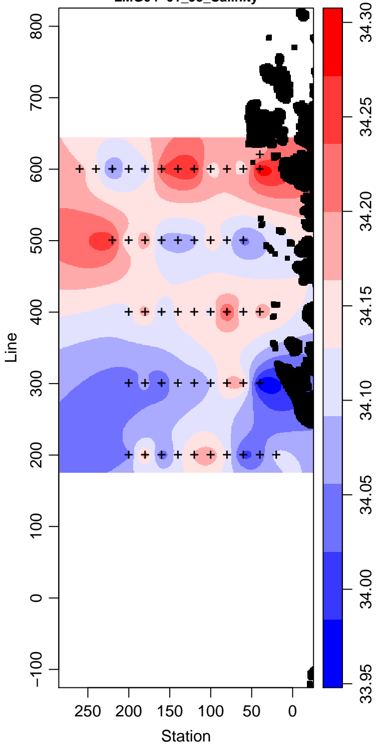
LMG04-01_95_Salinity
