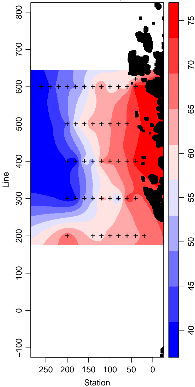
LMG04-01_35_Silicate \mu\text{ mol L}^{-1}
