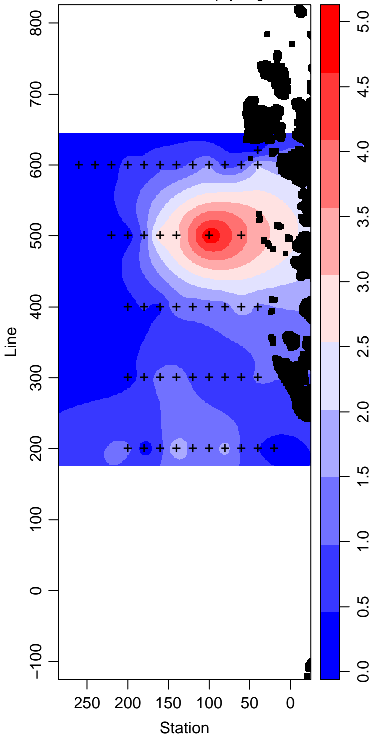
LMG05-01_15_Chlorophyll mg m -3
