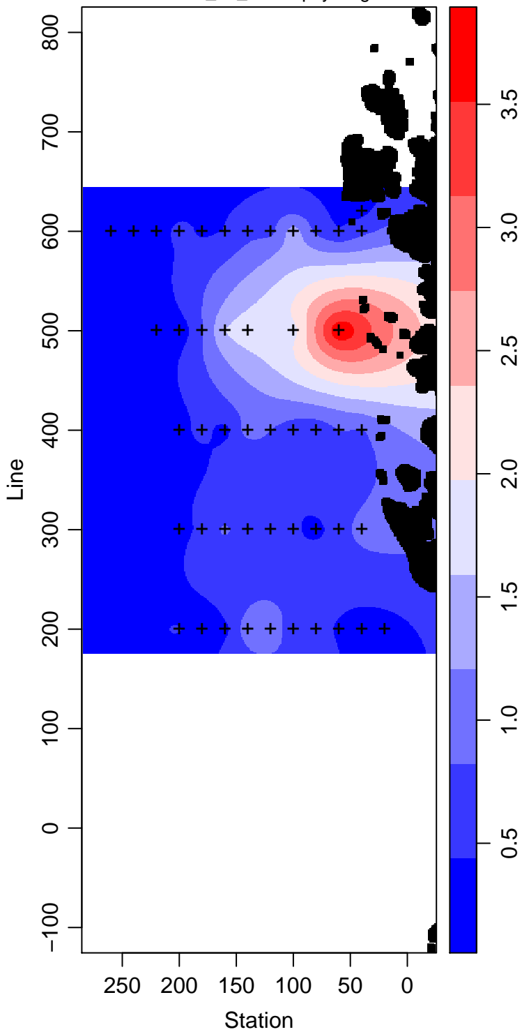
LMG05-01_25_Chlorophyll mg m -3
