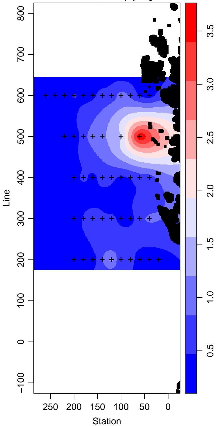
LMG05-01_30_Chlorophyll mg m -3
