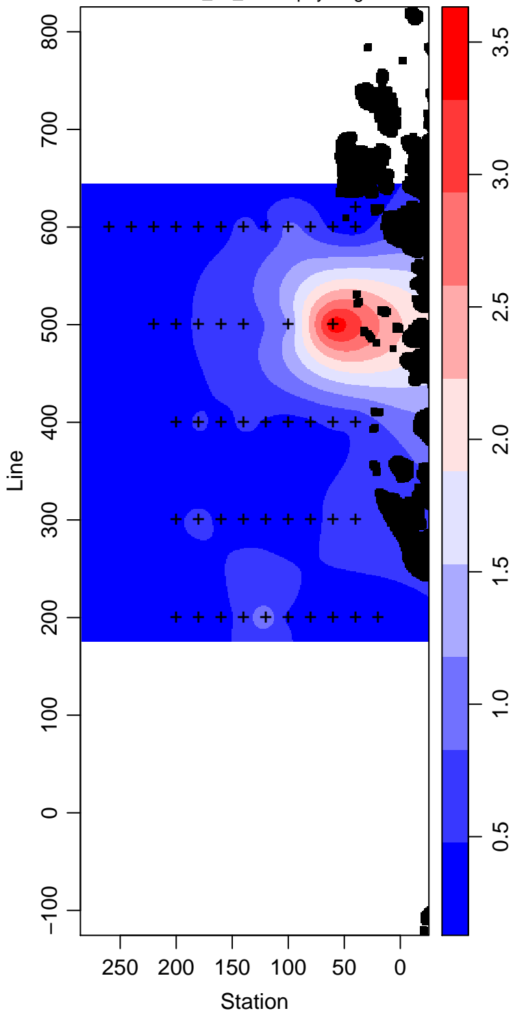
LMG05-01_35_Chlorophyll mg m -3
