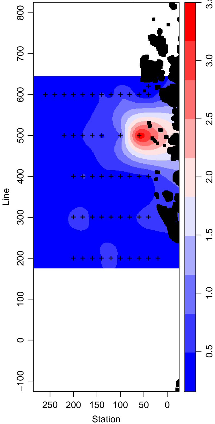
LMG05-01_40_Chlorophyll mg m -3
