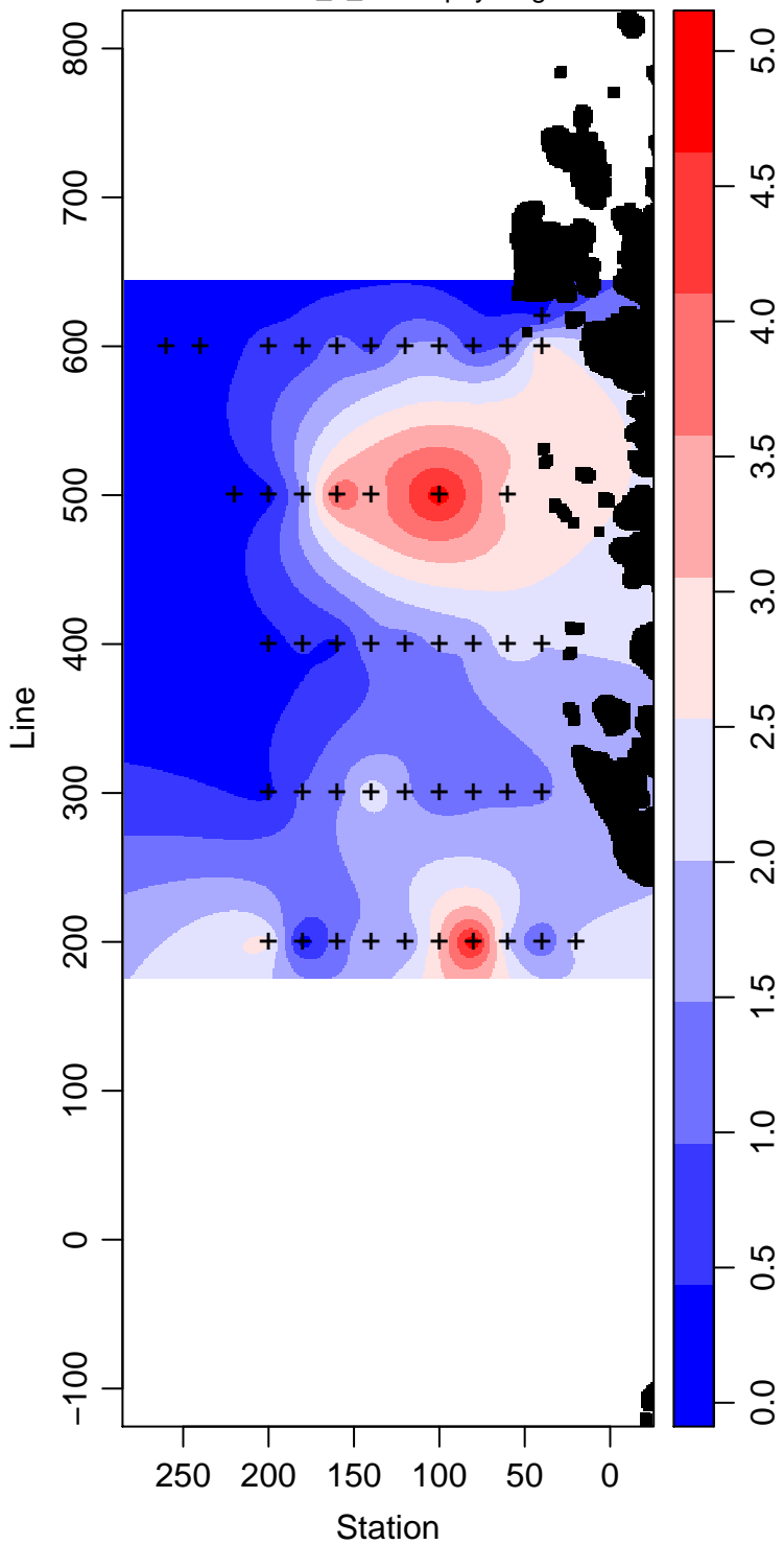
LMG05-01_5_Chlorophyll mg m -3
