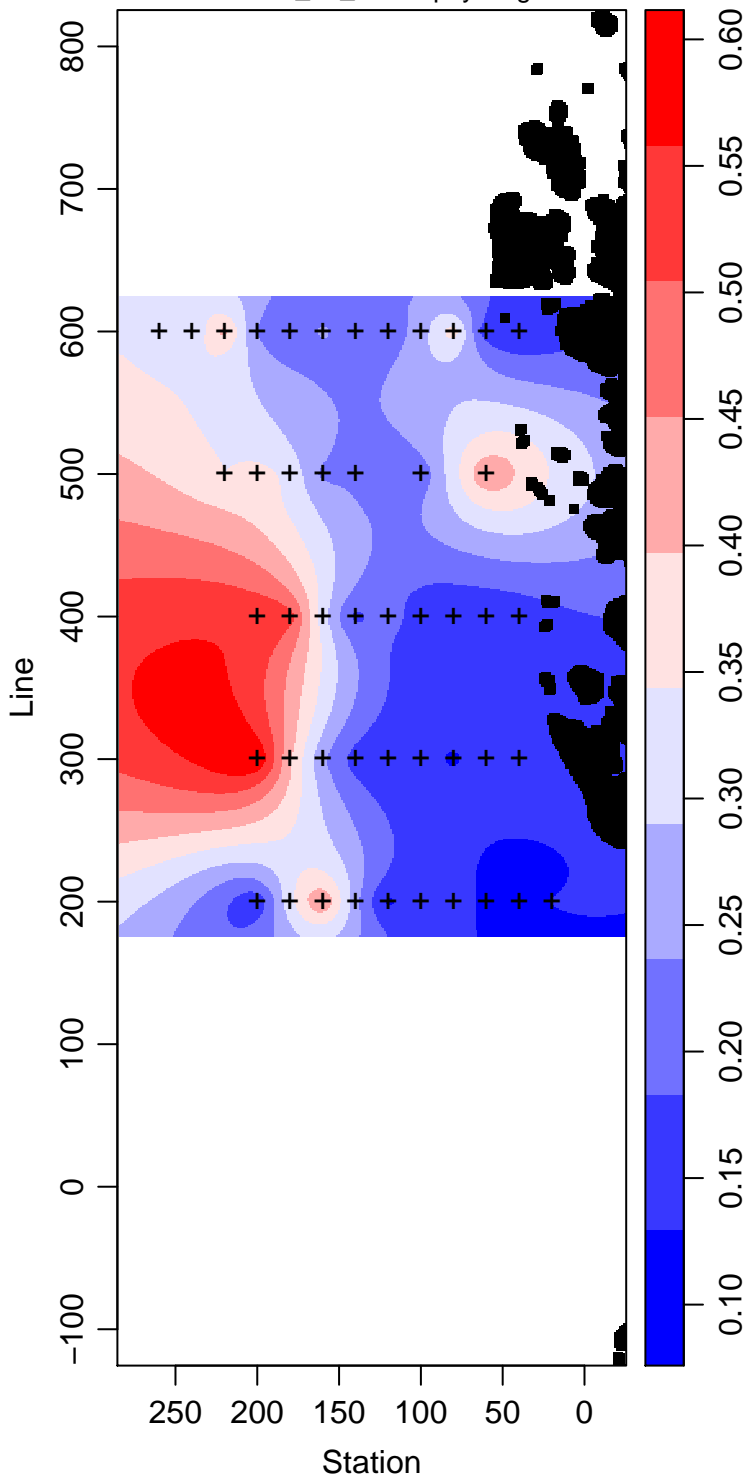
LMG05-01_70_Chlorophyll mg m -3
