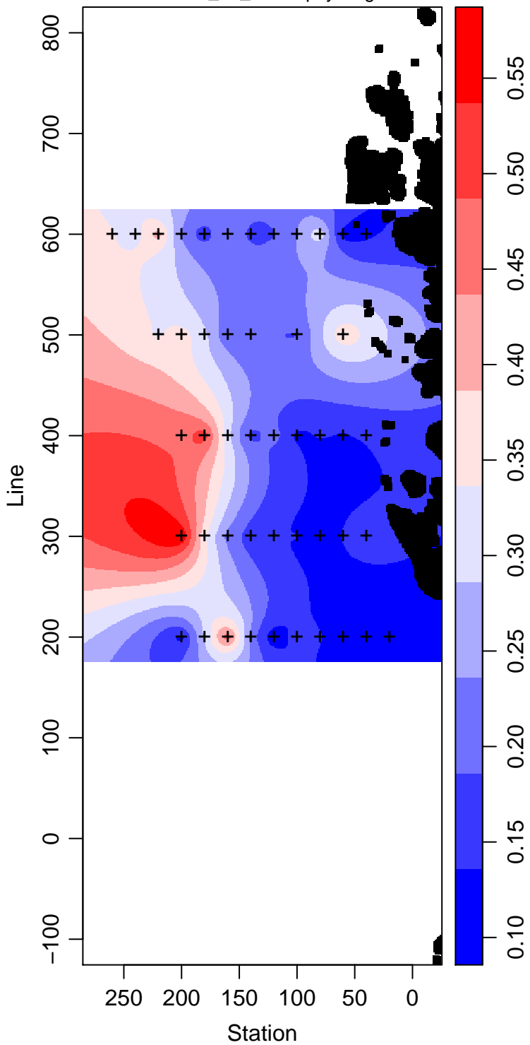
LMG05-01_75_Chlorophyll mg m -3
