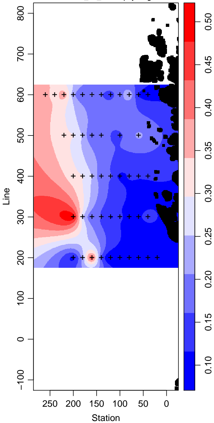
LMG05-01_85_Chlorophyll \text{mg m}^{-3}
