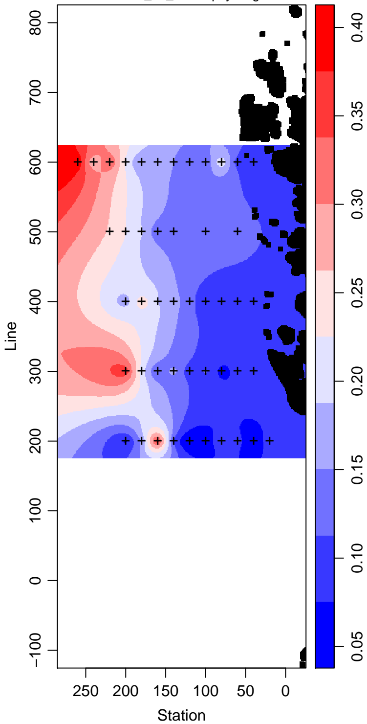
LMG05-01_95_Chlorophyll mg m -3
