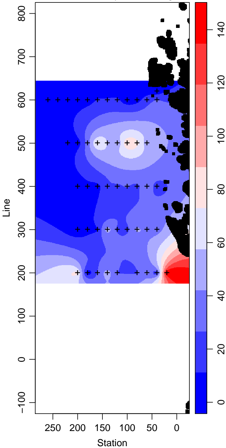
LMG05-01_1_Primary.Production mg m -3
