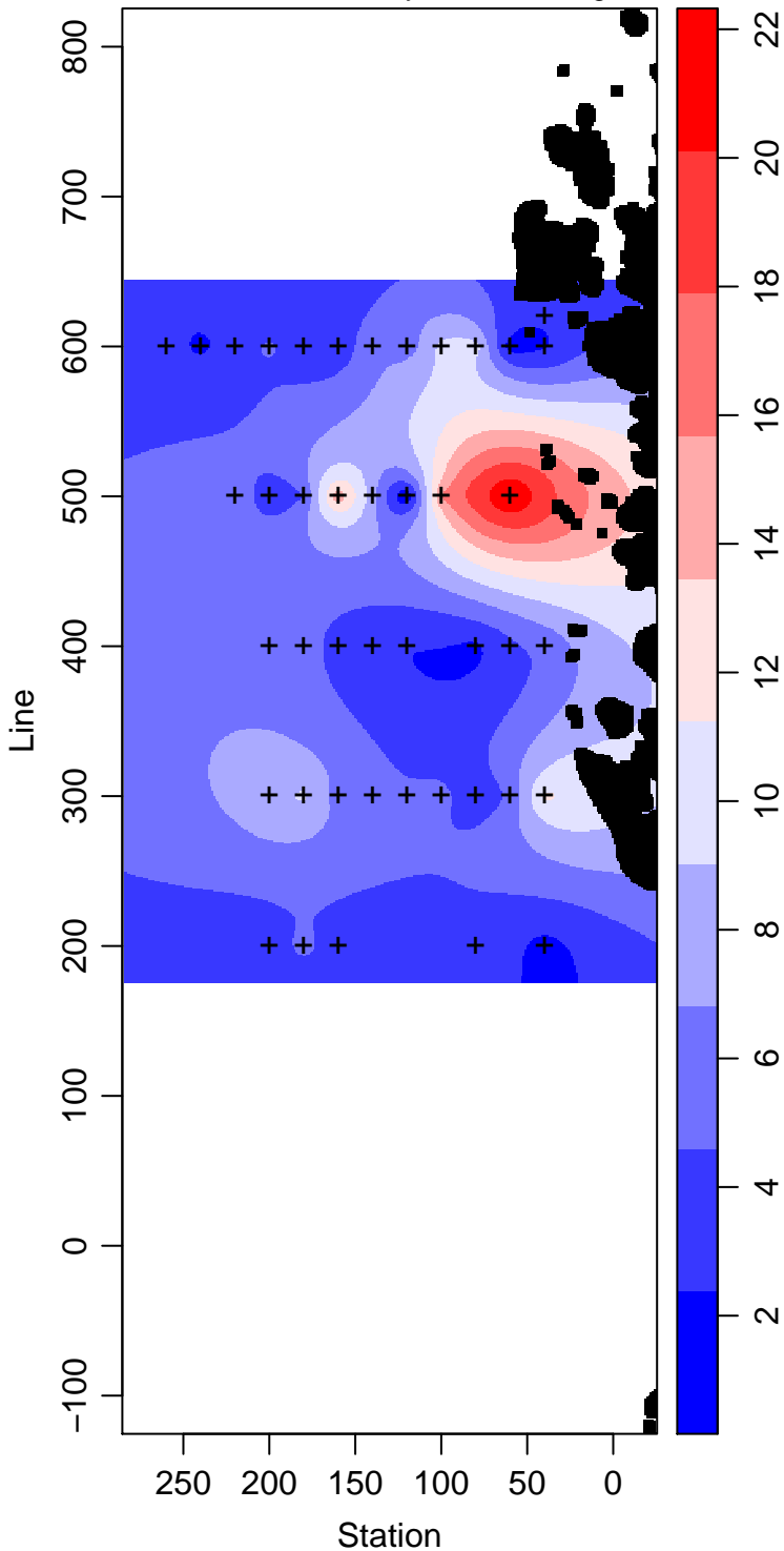
LMG05-01_35_Primary.Production mg m -3
