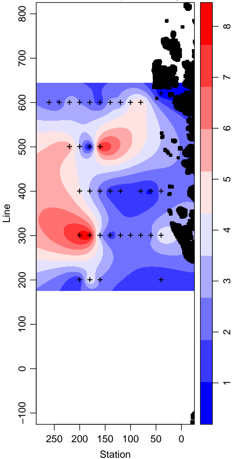
LMG05-01_55_Primary.Production mg m -3
