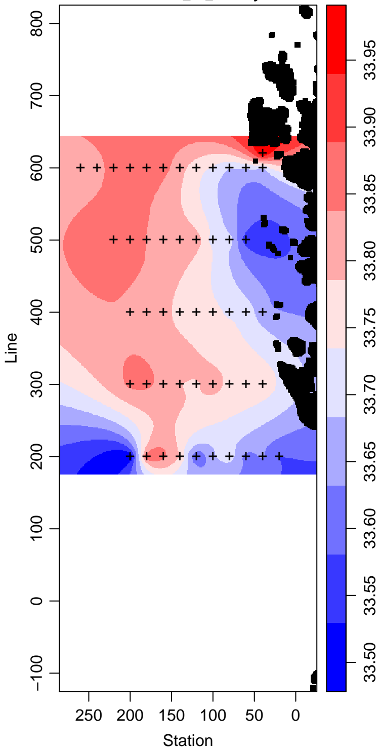
LMG05-01_35_Salinity
