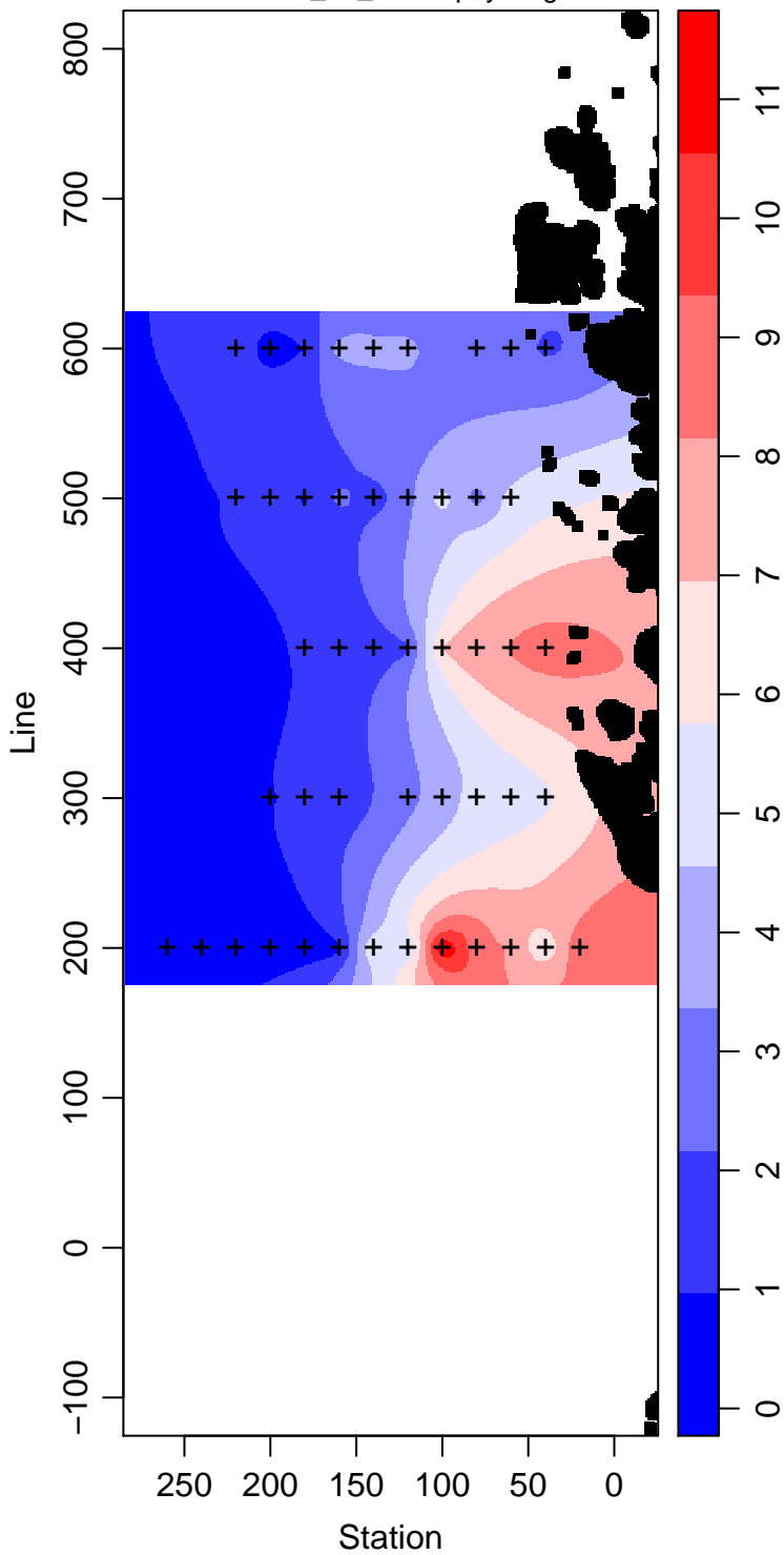
LMG06-01_10_Chlorophyll mg m -3
