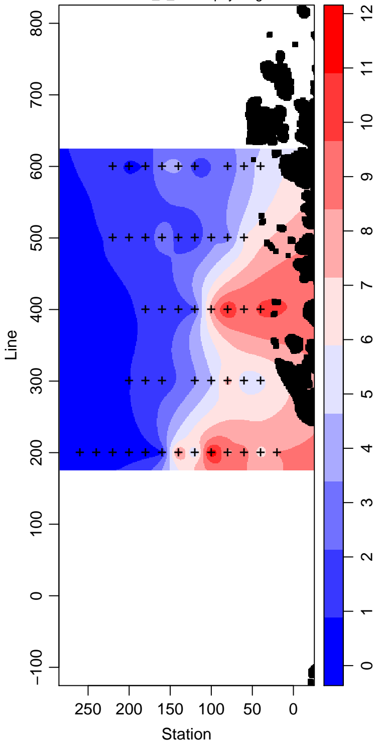
LMG06-01_1_Chlorophyll mg m -3
