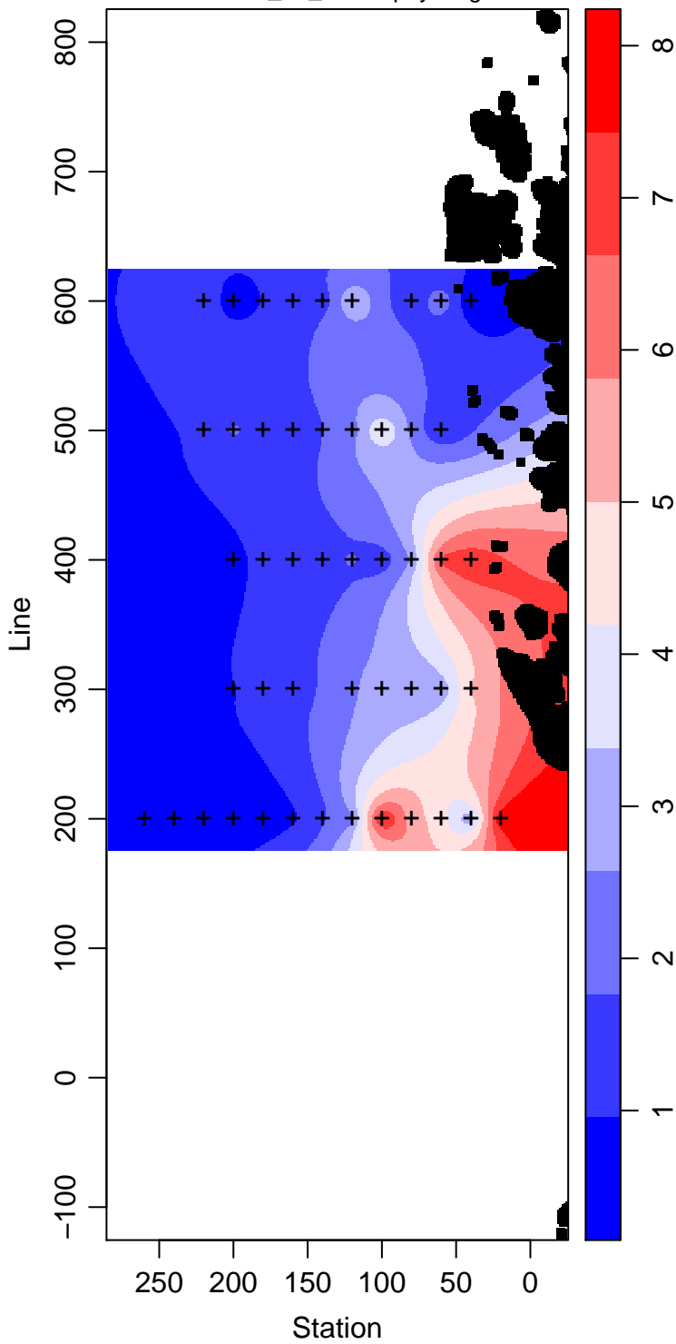
LMG06-01_25_Chlorophyll mg m -3
