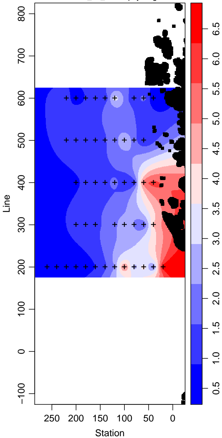
LMG06-01_30_Chlorophyll mg m -3
