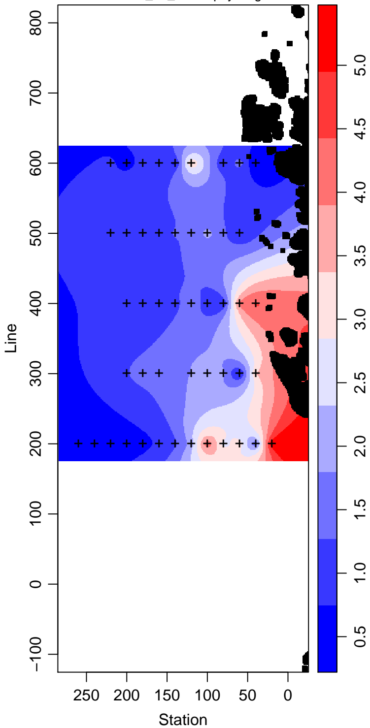
LMG06-01_35_Chlorophyll mg m -3
