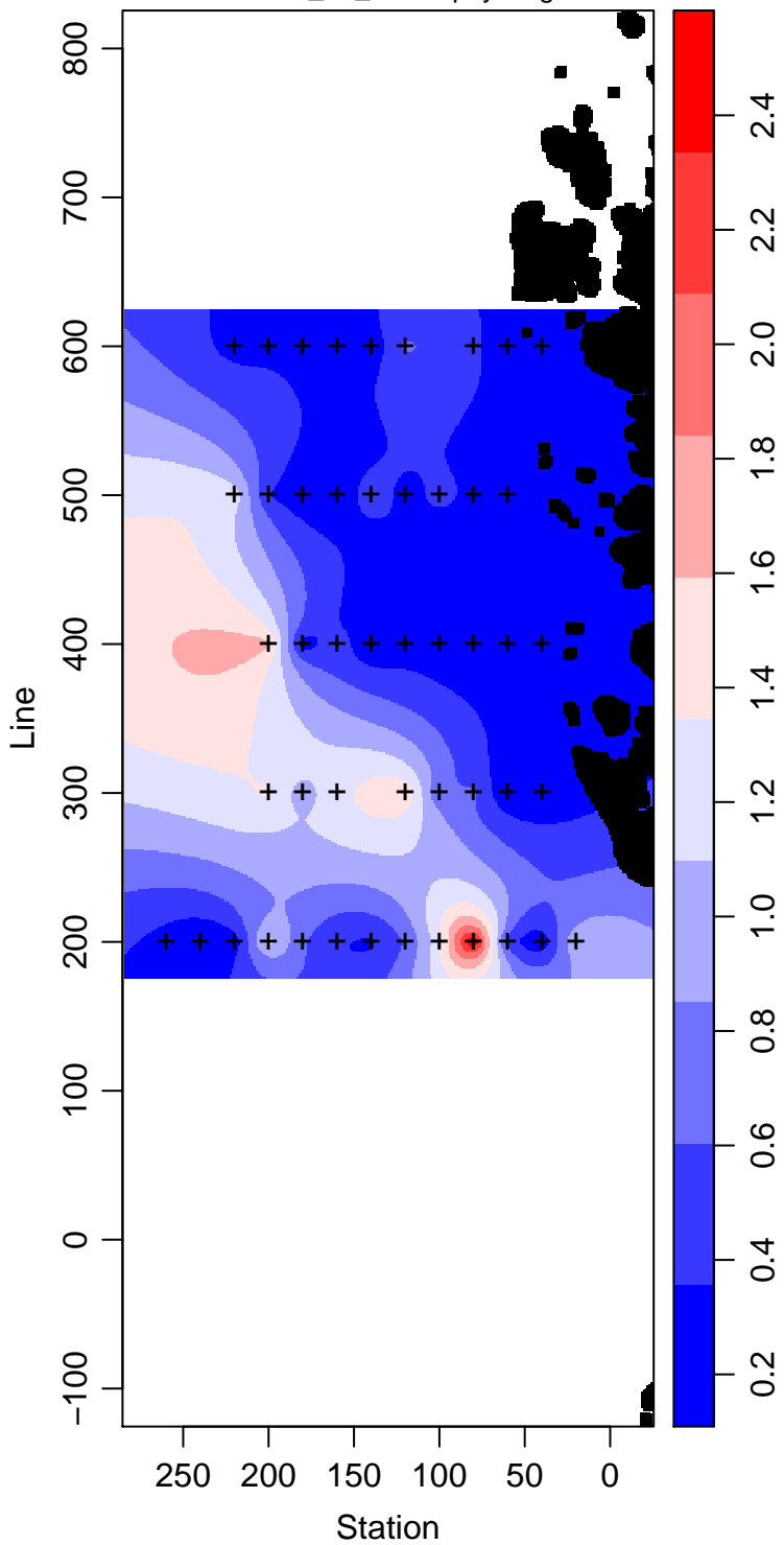
LMG06-01_60_Chlorophyll mg m -3
