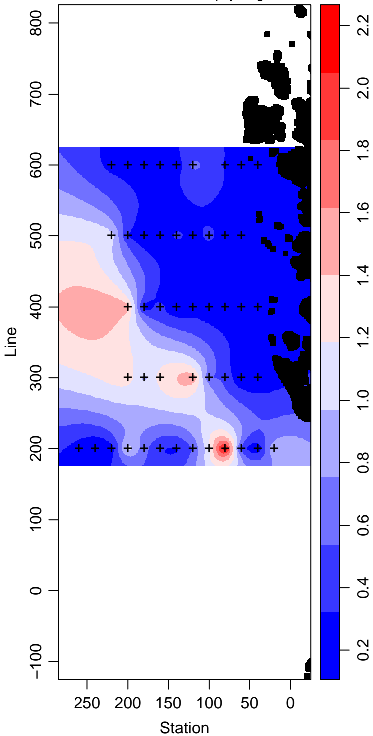
LMG06-01_65_Chlorophyll mg m -3
