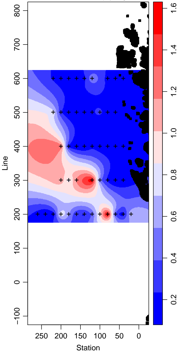
LMG06-01_75_Chlorophyll mg m -3
