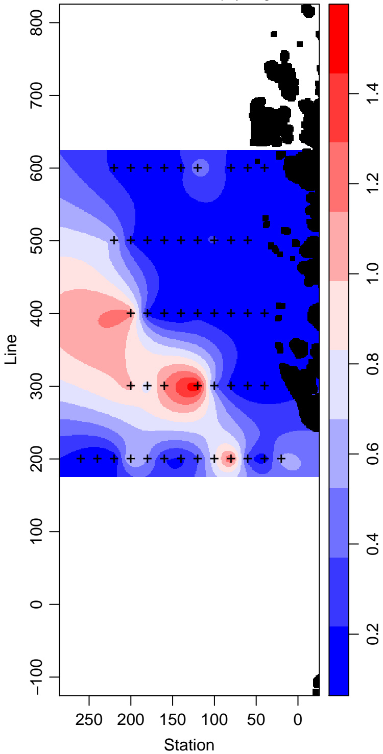
LMG06-01_80_Chlorophyll mg m -3
