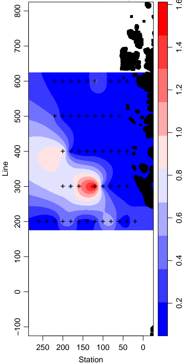
LMG06-01_90_Chlorophyll mg m -3
