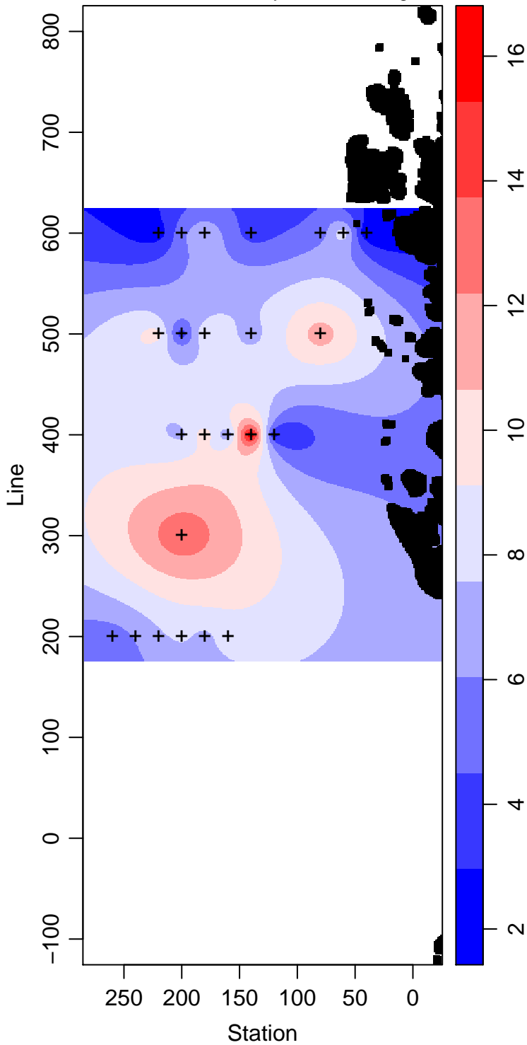
LMG06-01_40_Primary.Production mg m -3
