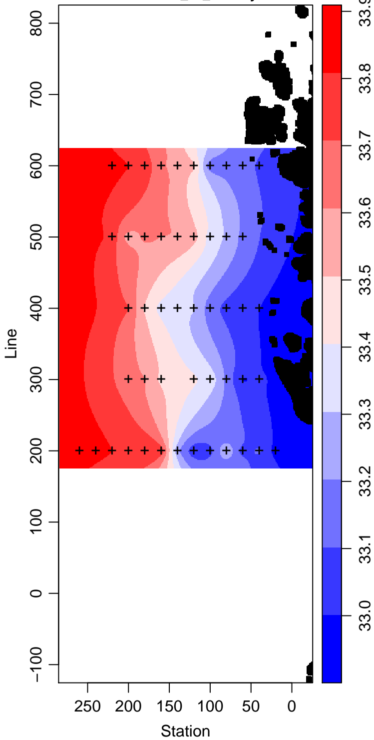
LMG06-01_10_Salinity
