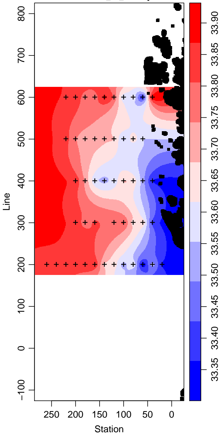
LMG06-01_35_Salinity
