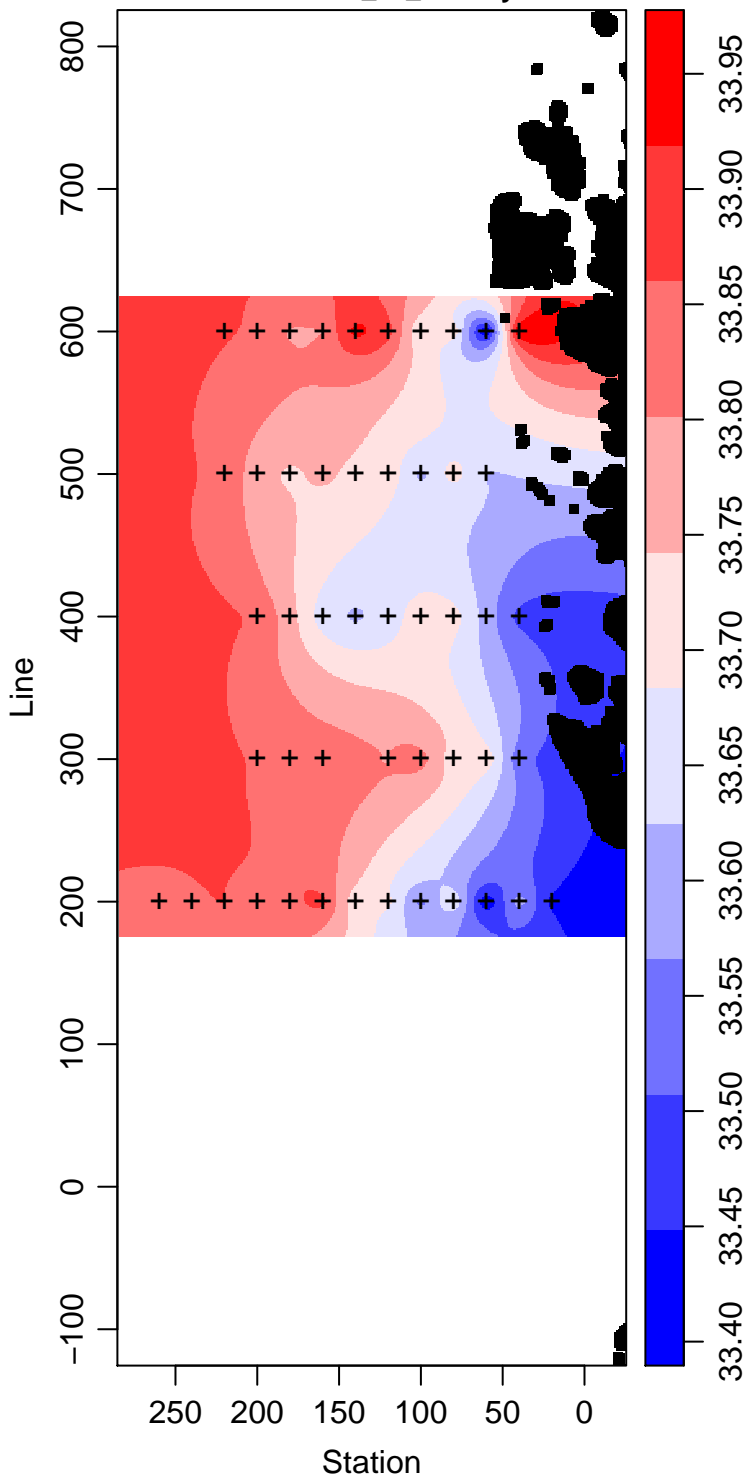
LMG06-01_40_Salinity
