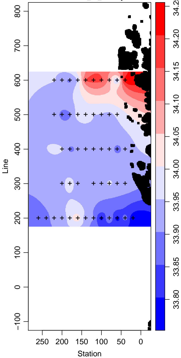
LMG06-01_70_Salinity
