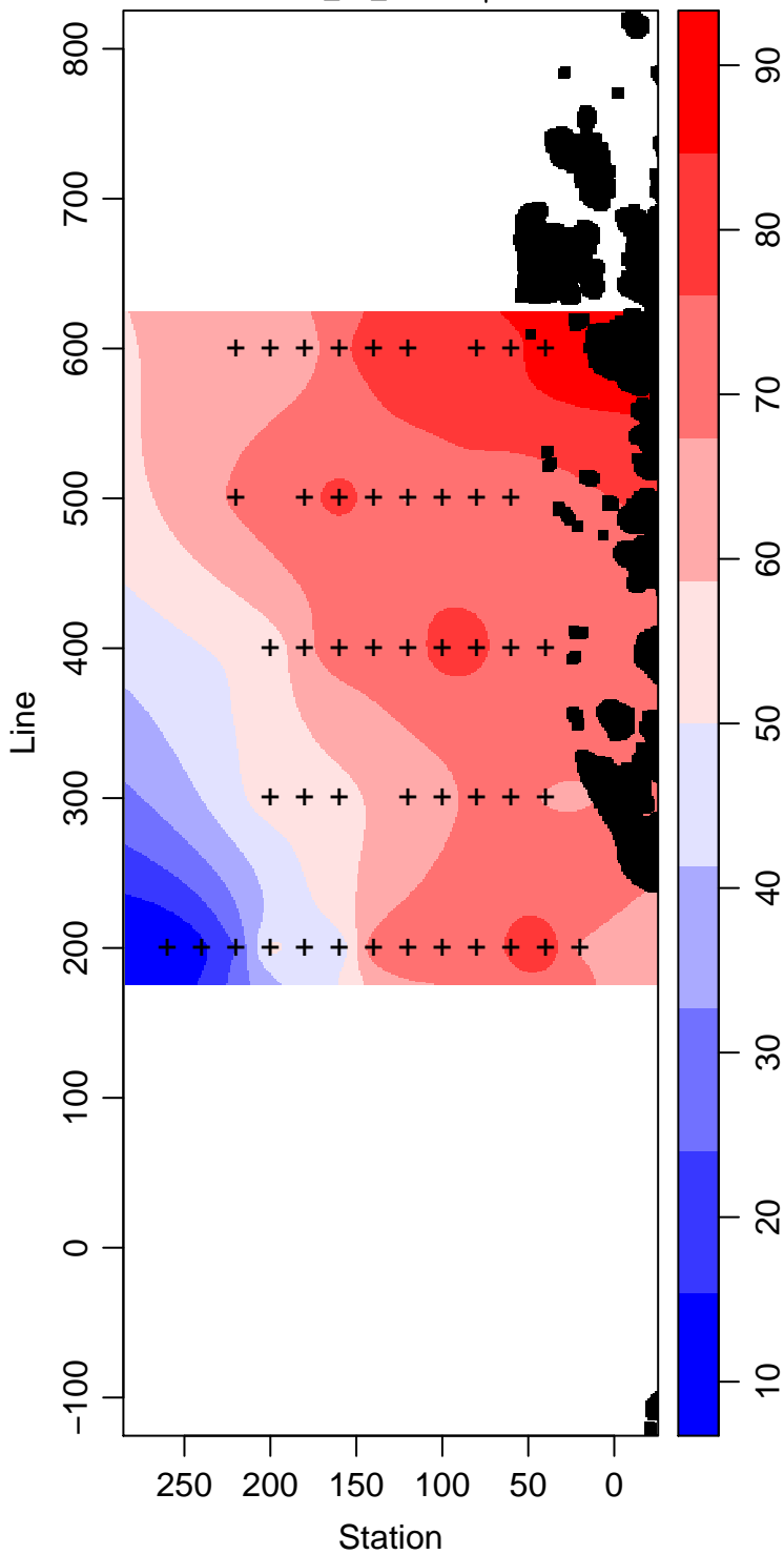
LMG06-01_35_Silicate \mu\text{ mol L}^{-1}
