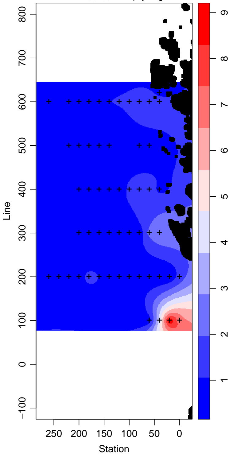
LMG07-01_25_Chlorophyll mg m -3
