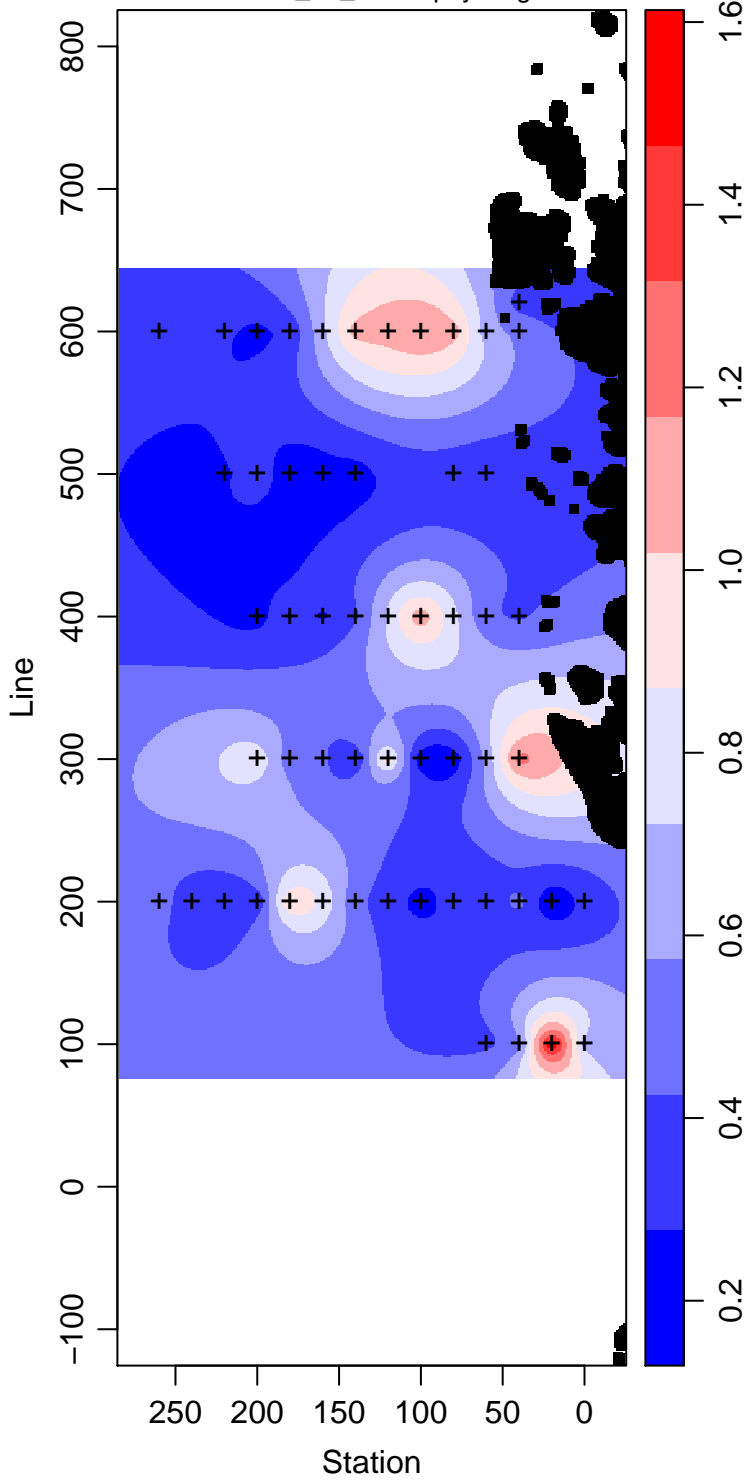
LMG07-01_50_Chlorophyll mg m -3
