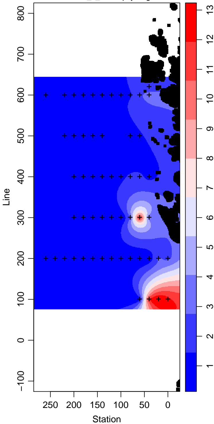
LMG07-01_5_Chlorophyll mg m -3
