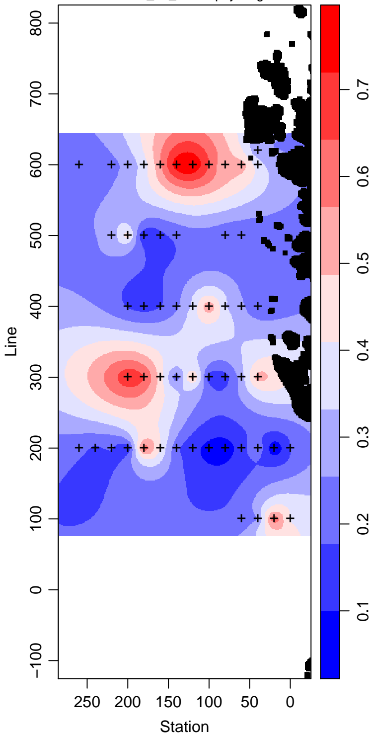
LMG07-01_65_Chlorophyll mg m -3
