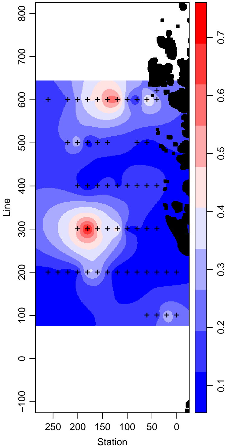
LMG07-01_75_Chlorophyll mg m -3
