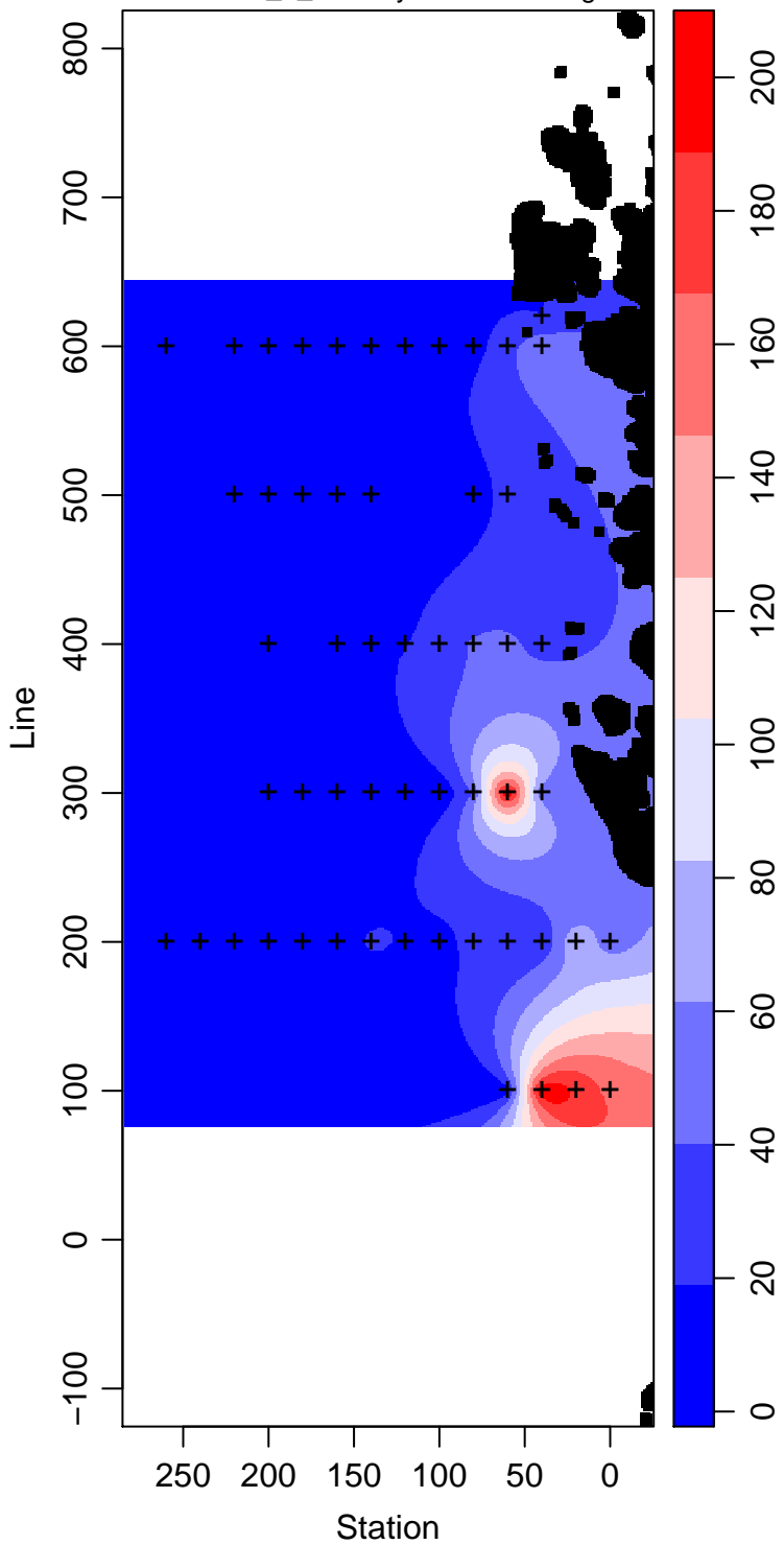
LMG07-01_1_Primary.Production mg m -3
