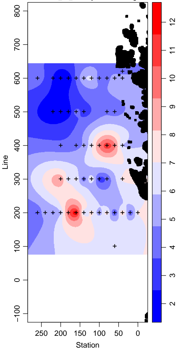
LMG07-01_40_Primary.Production mg m -3
