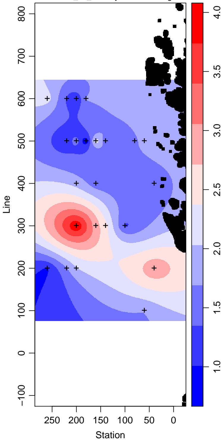
LMG07-01_65_Primary.Production mg m -3
