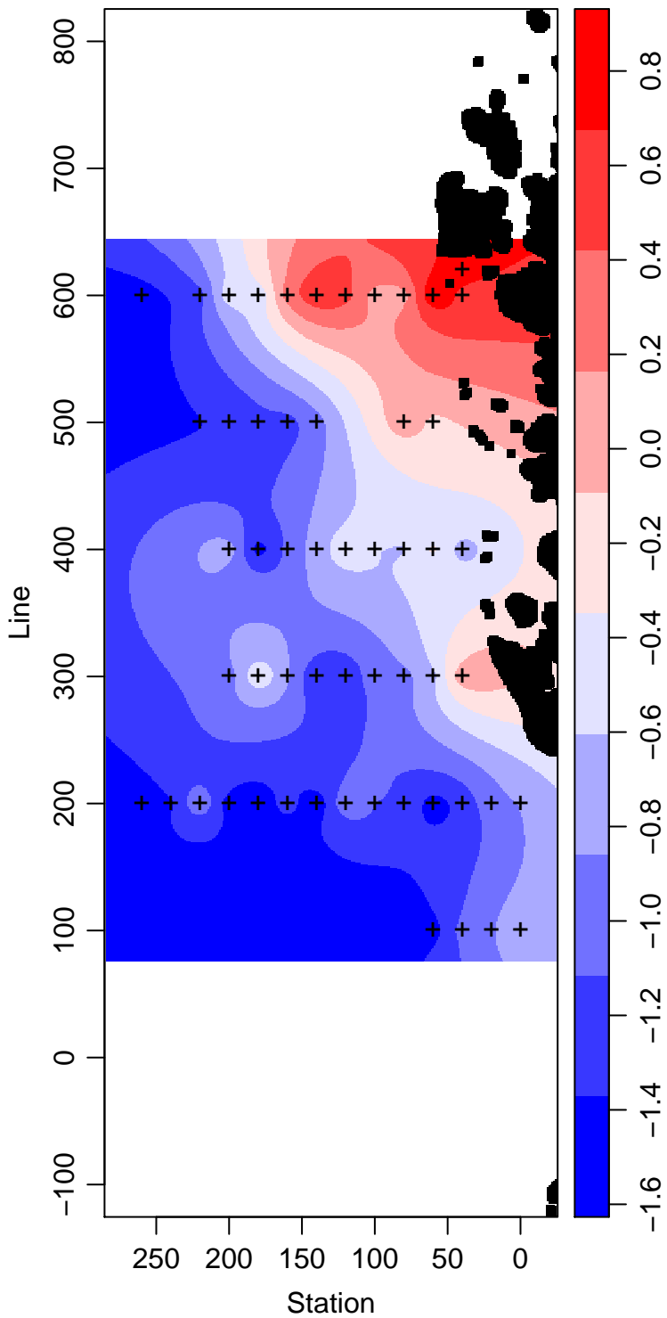
LMG07-01_70_Temperature ° Celsius
