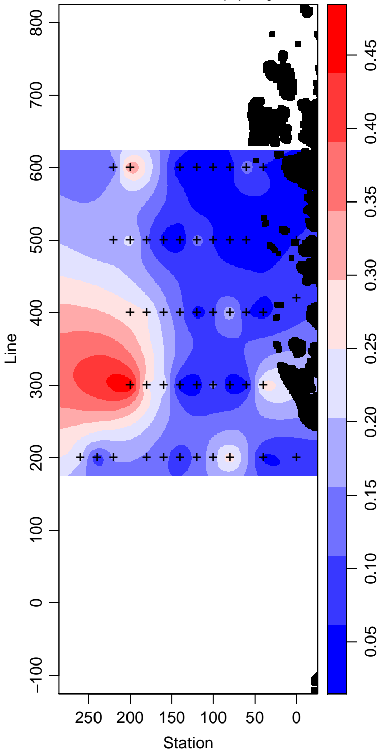
LMG08-01_100_Chlorophyll mg m -3
