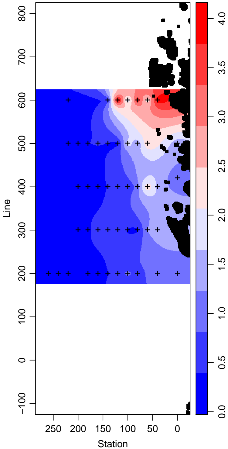
LMG08-01_10_Chlorophyll mg m -3
